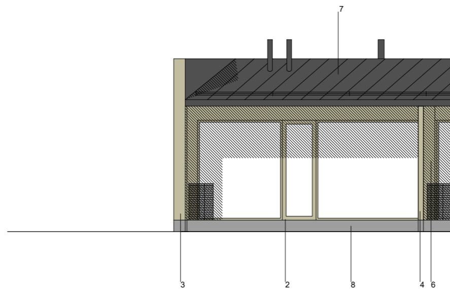
Julkisivu etelään
