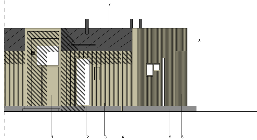
Julkisivu pohjoiseen
