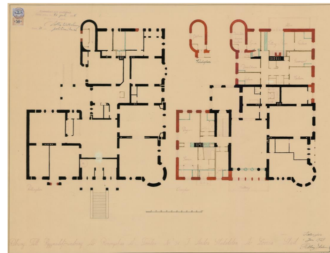
Kuva 12. Pohjapiirroksat 1. ja 2. krs. Ensimmäisen kerroksen pohjapiirros on pysynyt lähes samana, vain eteläjulkisivun kulmikas erkkeriäihe on poistettu. Pääsisäänkäynnin portaat ovat suunnitelmassa suorat. Toisen kerroksen muutokset ovat huomattavat (kts. kuva 13).
