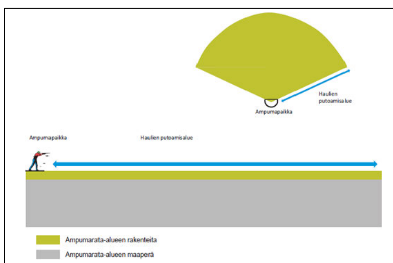
Kuva 13. Haulikoratojen ratarakenne (Ympäristöministeriö, 2012).
