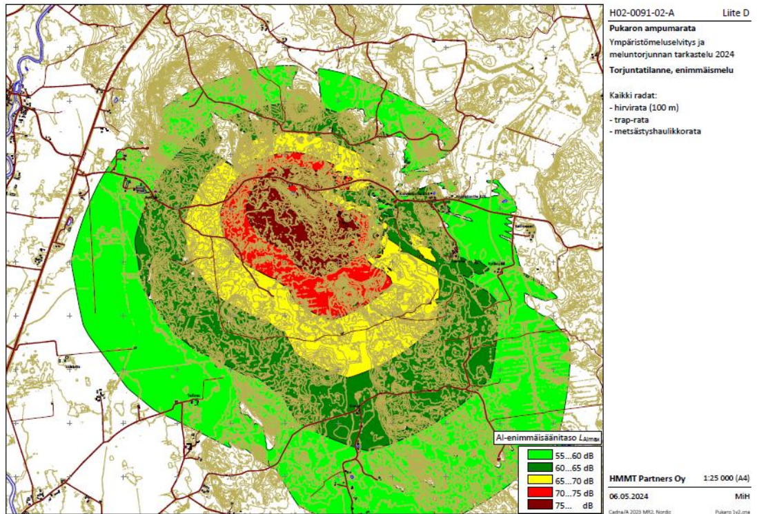
Kuva 11 Torjuntatilanne, enimmäismelu
