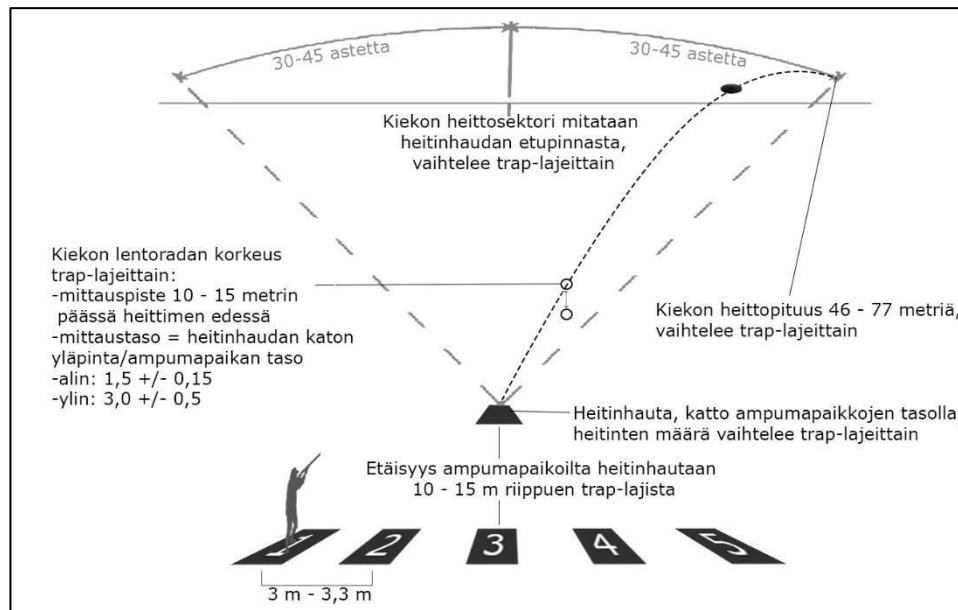
Kuva 14. Trap-radan periaatepiirros. (Pelkonen, 2022)
