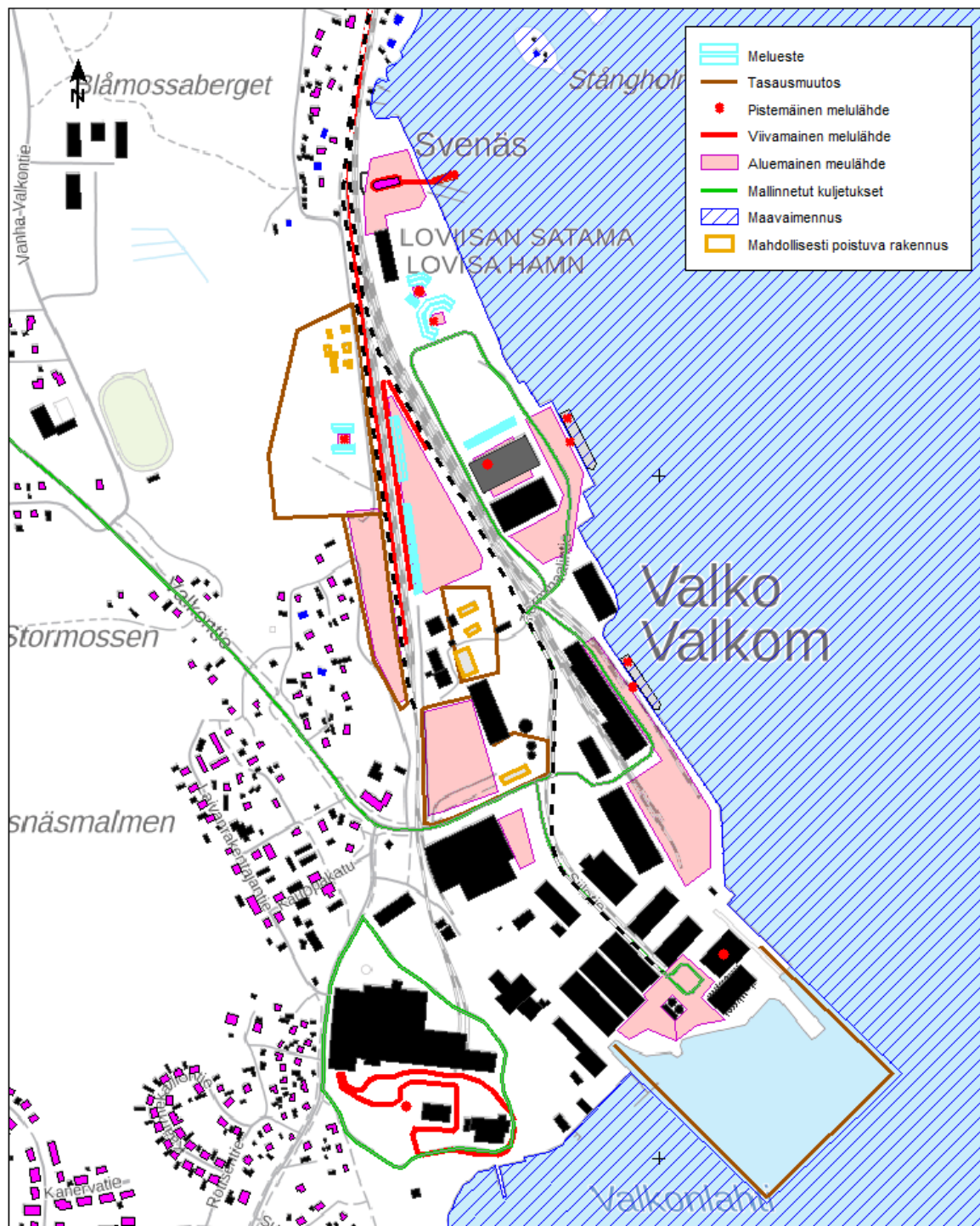
Kuva 3. Satama-alueen melulähteet ja tasausmuutosalueet kasvuennustetilanteessa
