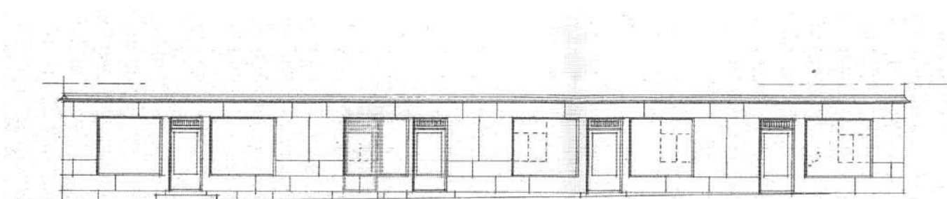
FASAD MOT ALEXANDERSGATAN
