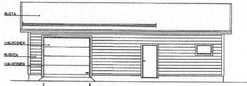
JULKISIVU PÖHJOISEEN
