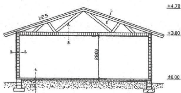
LEIKKAUS A-A
