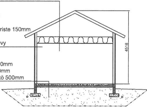
Leikkaus
